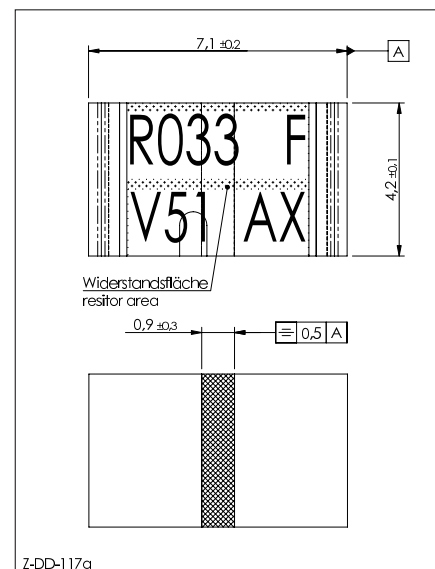
Bauform / Size 2817
