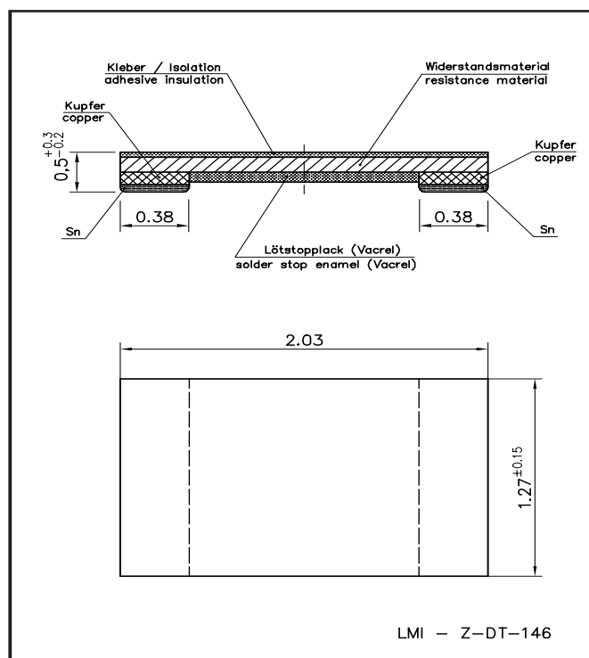
Bauform/Size 0805
